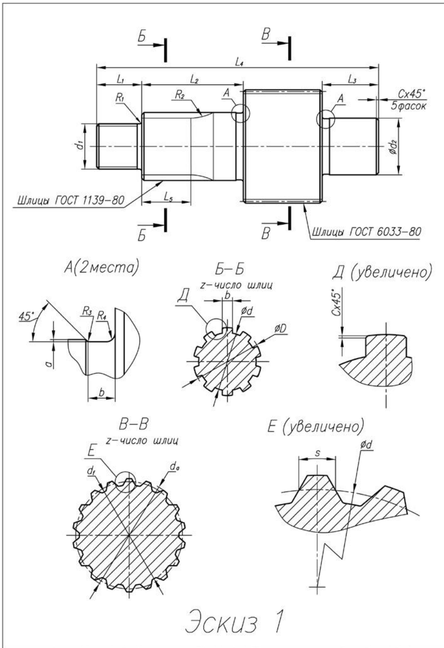
Рисунок 1 – Эскизы вала и шестерни Таблица 3
