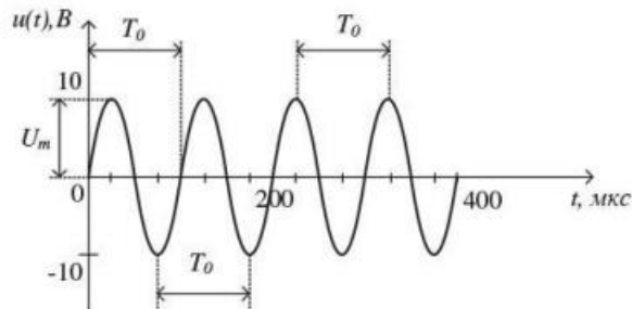
Рис. 1.1. Гармонический сигнал
