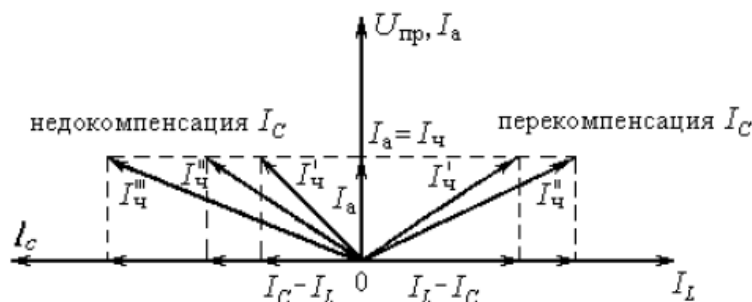
Рис. 12. Векторные диаграммы компенсации емкостного тока
