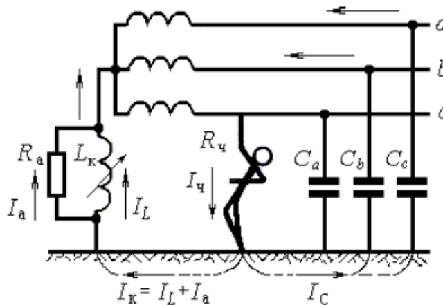
Рис. 11. Схема компенсации емкостного тока: L_K – компенсирующая катушка индуктивности; R_a – активное сопротивление катушки
