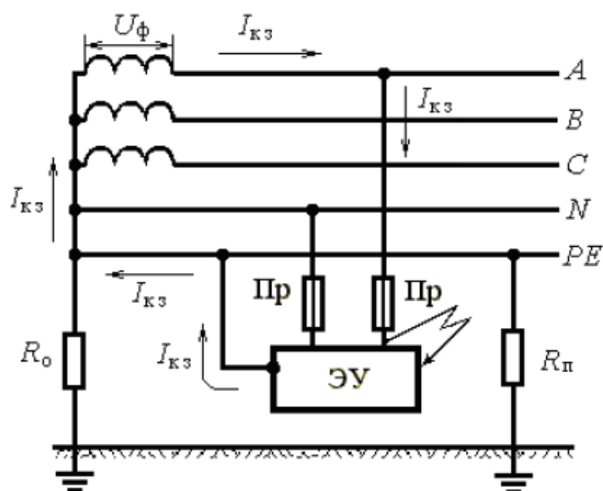
Рис. 3. Принципиальная схема зануления
