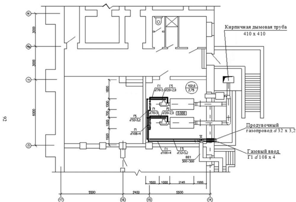
Рис. 1. План котельной административного здания
