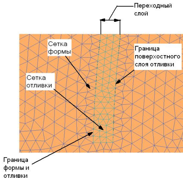
Рисунок 2. Разновидности конечно-элементной сетки.
