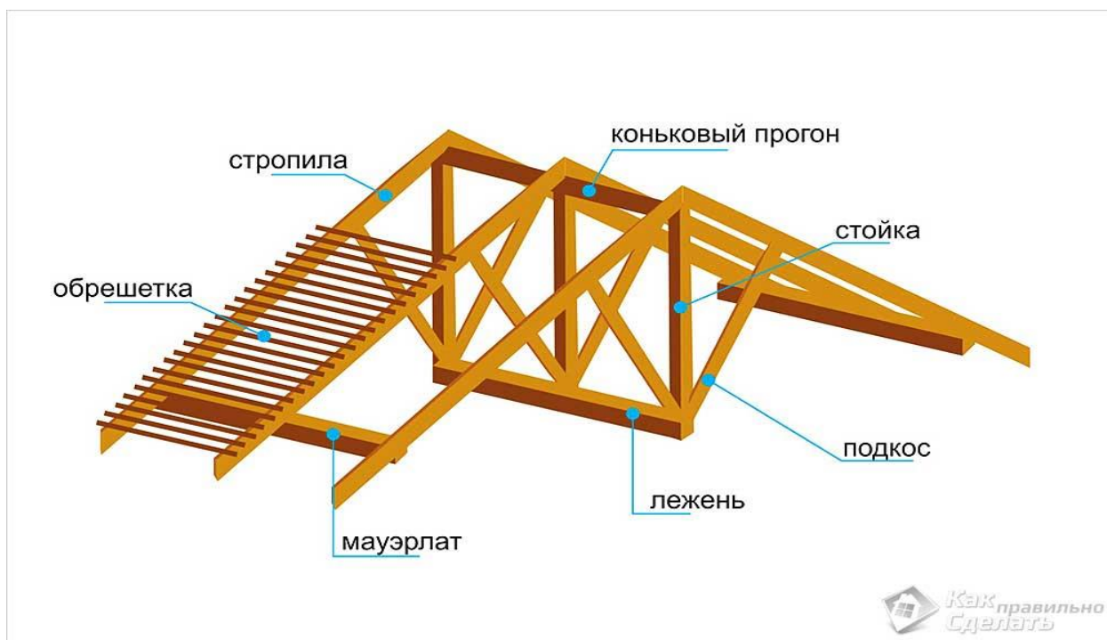
Рисунок 4.4 - Элементы стропильной системы
