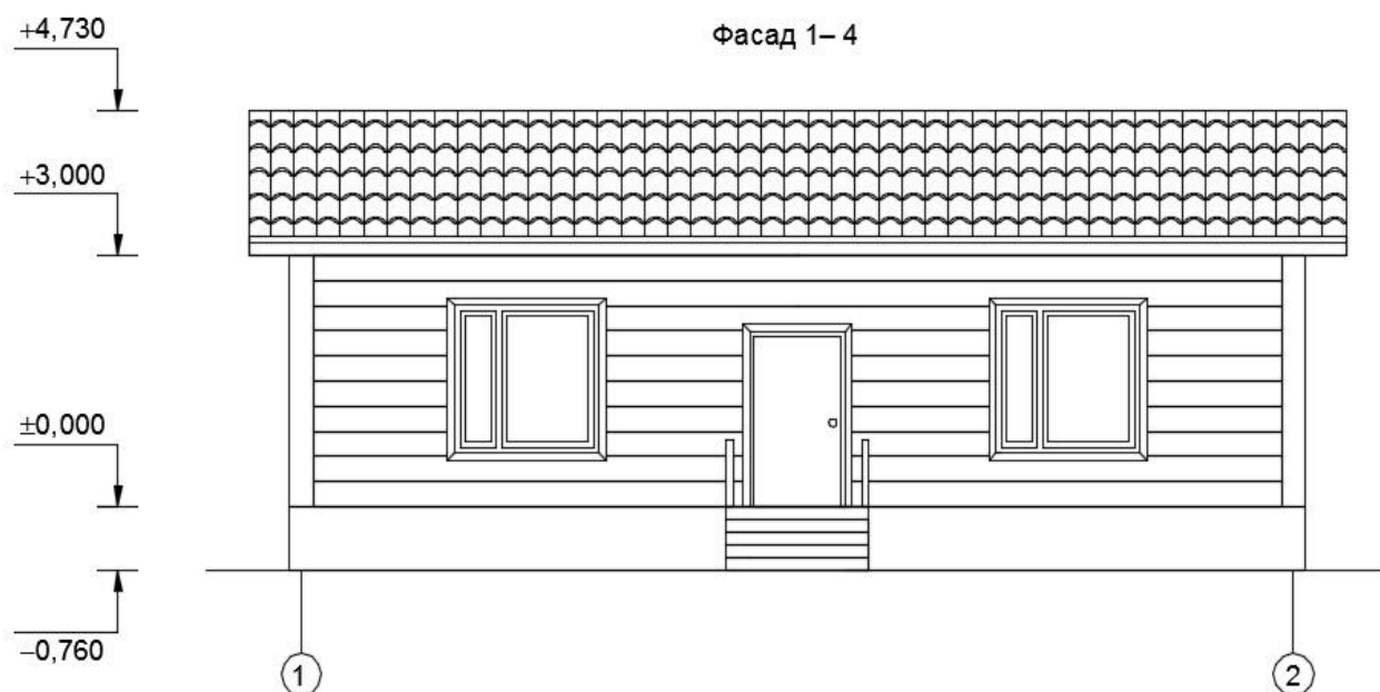
Рисунок 2.2 - Фасад книгохранилища
