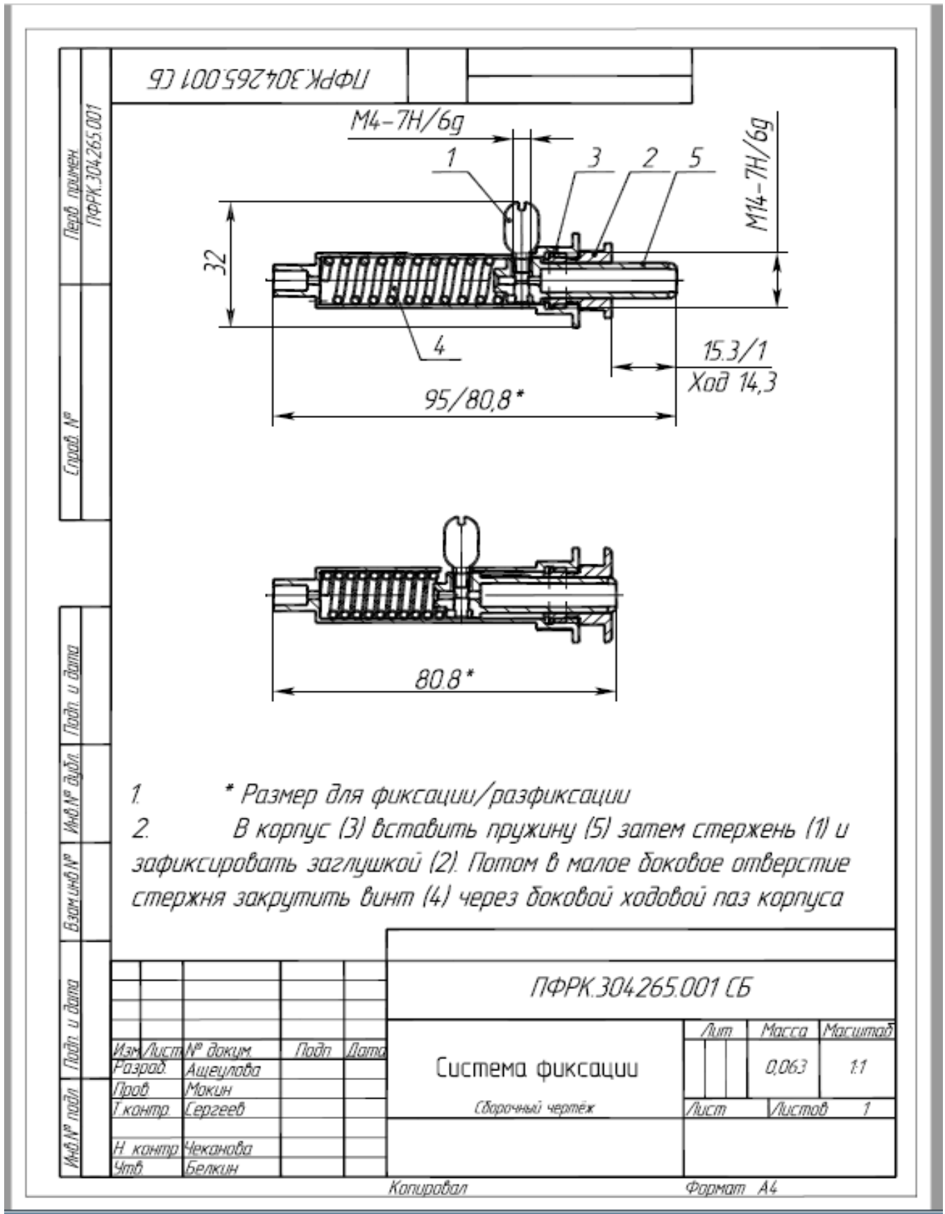
Пример Сборочные чертеж
