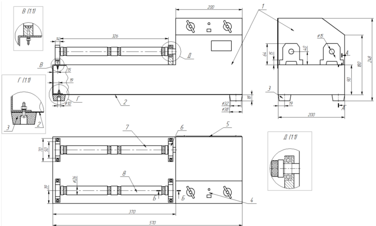
Рисунок 4. Галтовка барабанного типа
