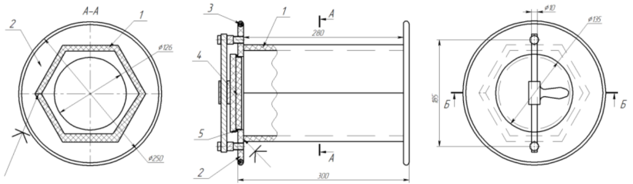
Рисунок 5. Галтовочный барабан.
