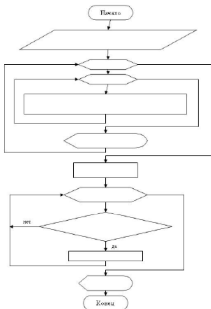
Рис.2.6. Блок-схема
