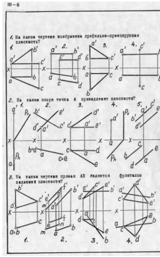
№3 Тема: Принадлежность точки прямой и плоскости
