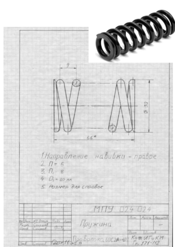
– Эскиз пружины
