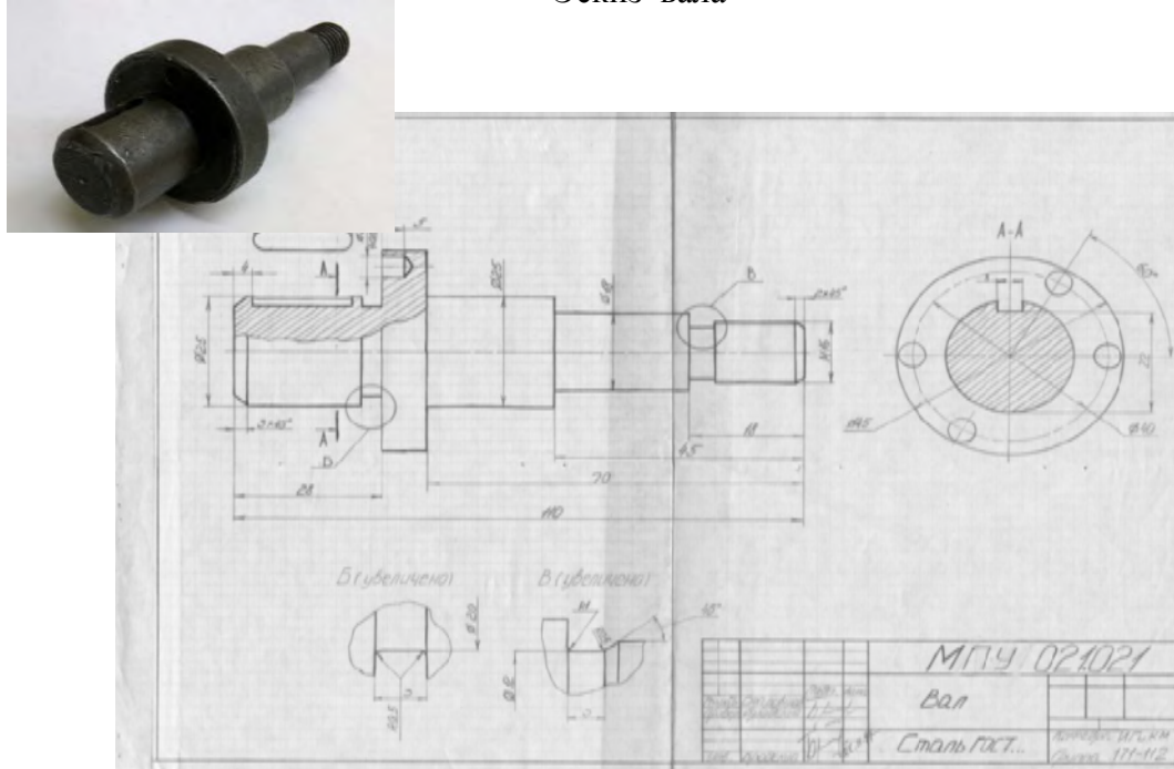
– Эскиз вала
