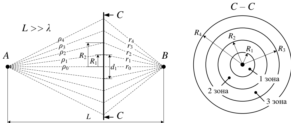
Рис. 2. Построение зон Френеля на плоскости
