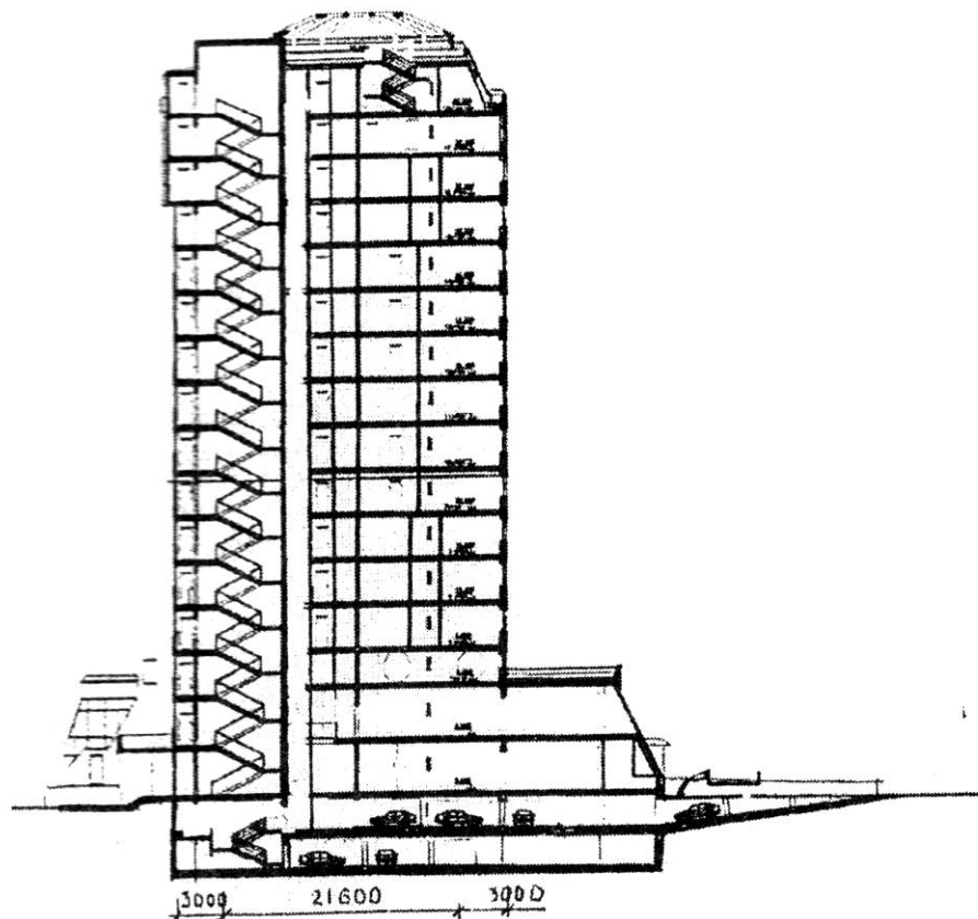
Разрез 1-1
