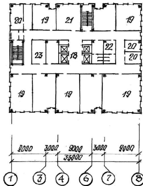
План типового этажа
