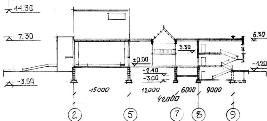
Разрез А-А
